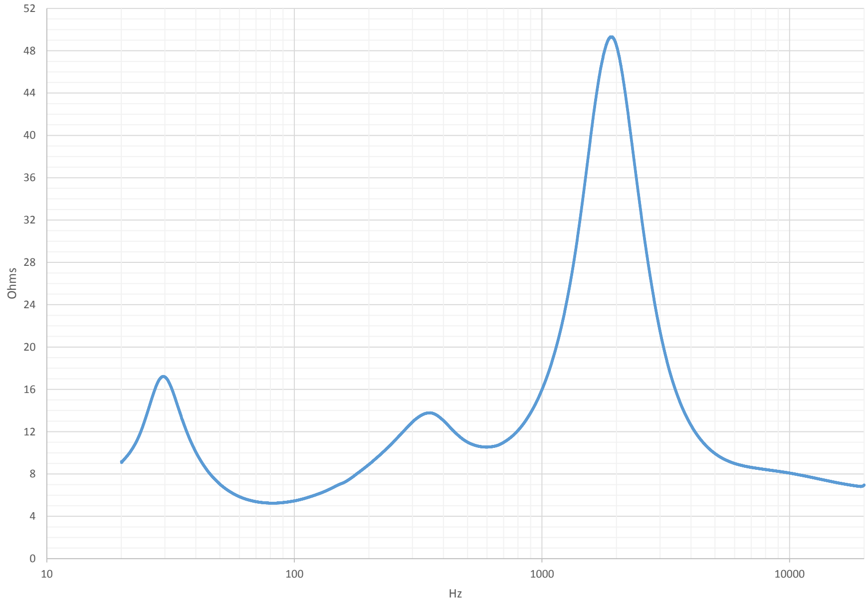
B&W 801 Impedance
